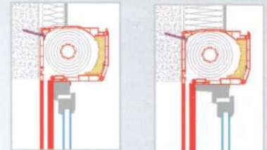
Pose en applique isolation 100 mm
