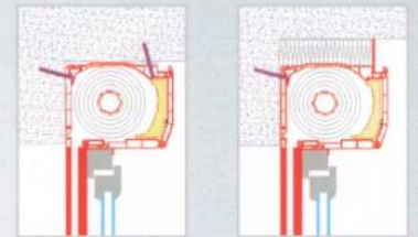
Pose en applique sous dalle
